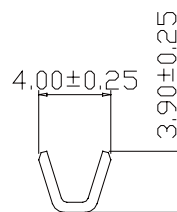
SEC: A-A
